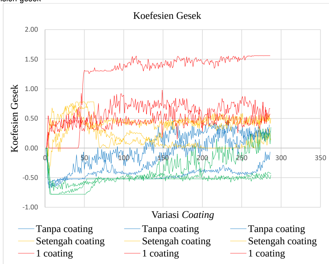
Gambar 25. Grafik perbandingan koefisien gesek
