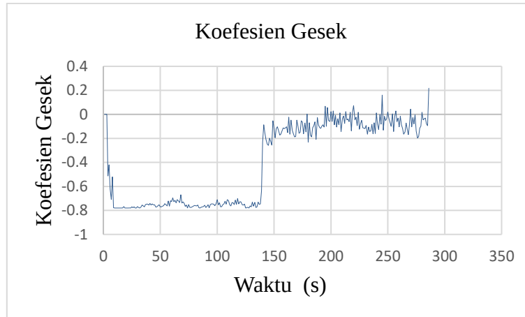
Gambar 14. Grafik koefisien gesek satu coating pengujian kedua.
