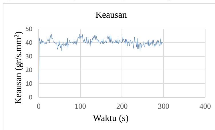
Gambar 18. Grafik keausan 1 coating pengujian ketiga.
