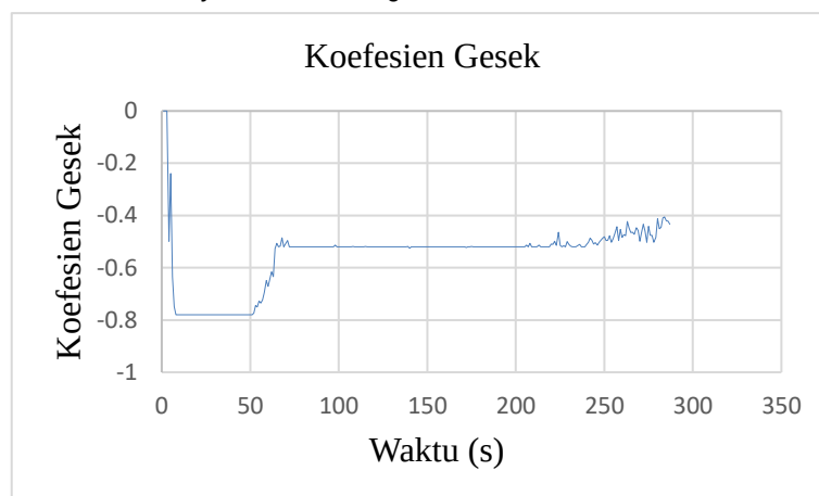
Gambar 20. Grafik Koefisien gesek 2 coating pengujian kedua.
