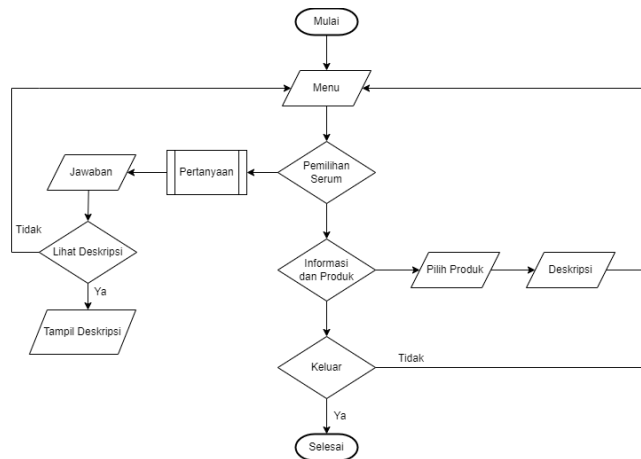
Gambar 4. Tampilan Flowchart Menu Utama
