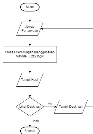
Gambar 5 Tampilan Flowchart Menu Pemilihan Serum
