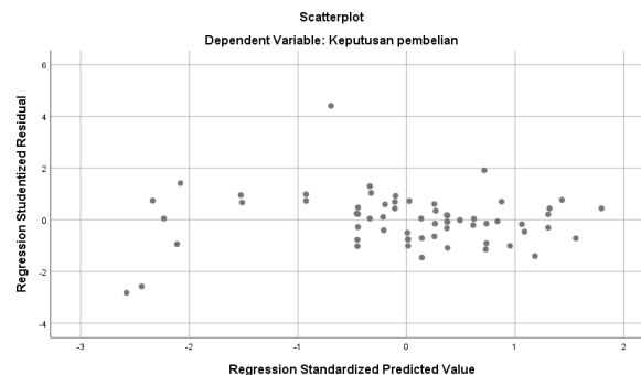
Gambar 2 Grafik Scatterplot
